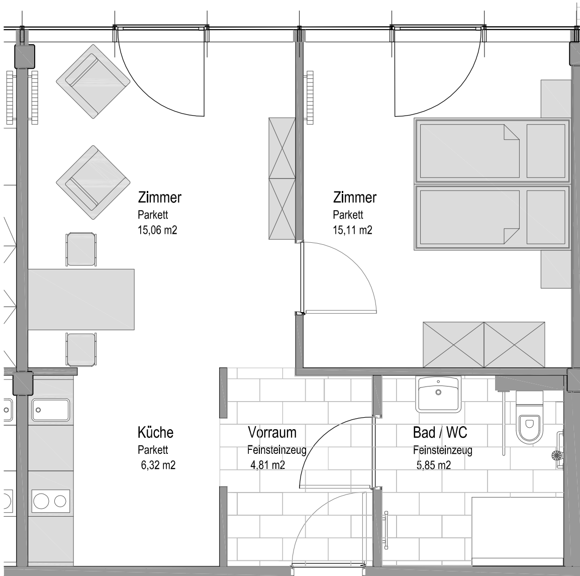
Grundriss M 1:50
