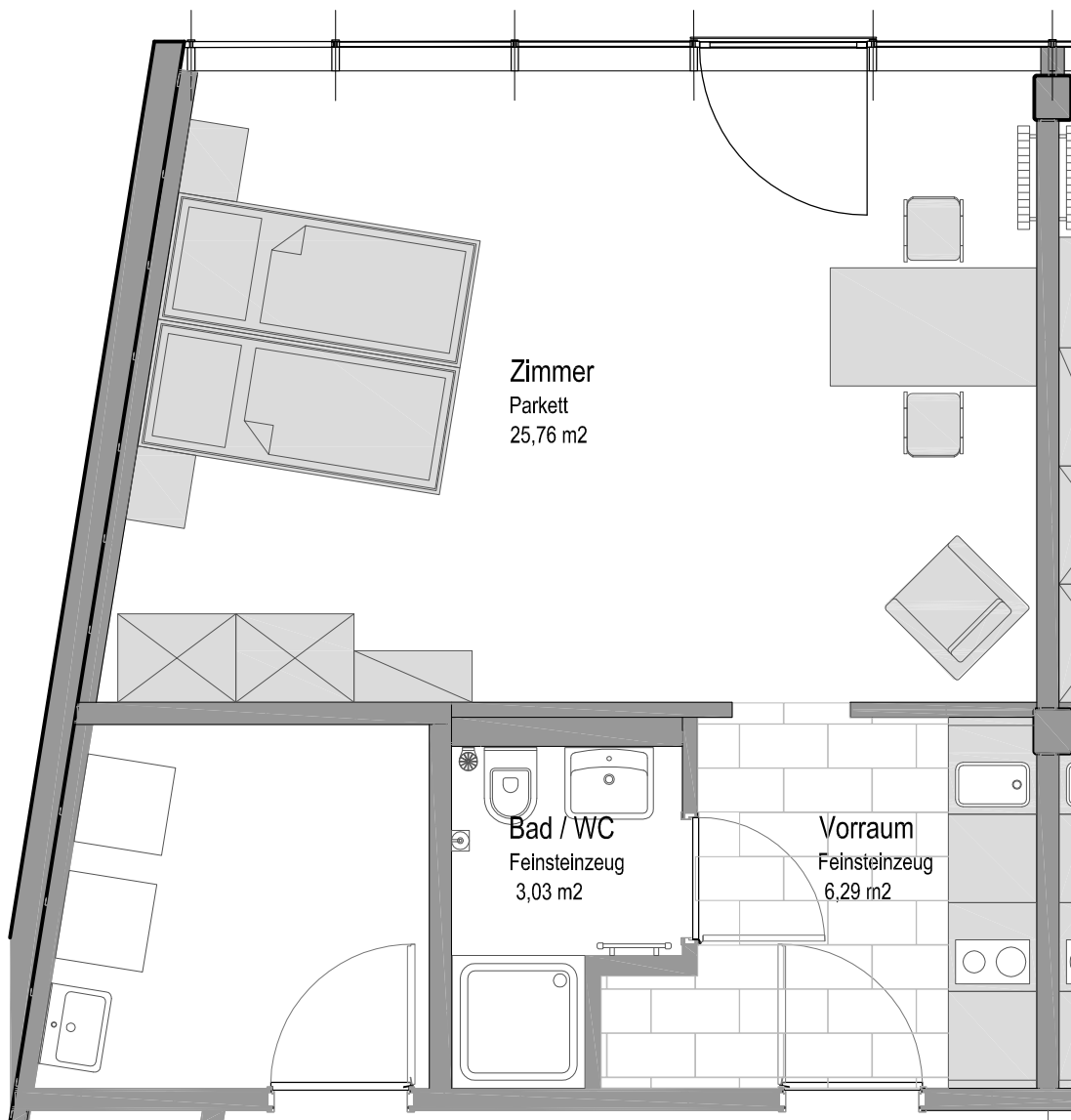
Grundriss M 1:50
