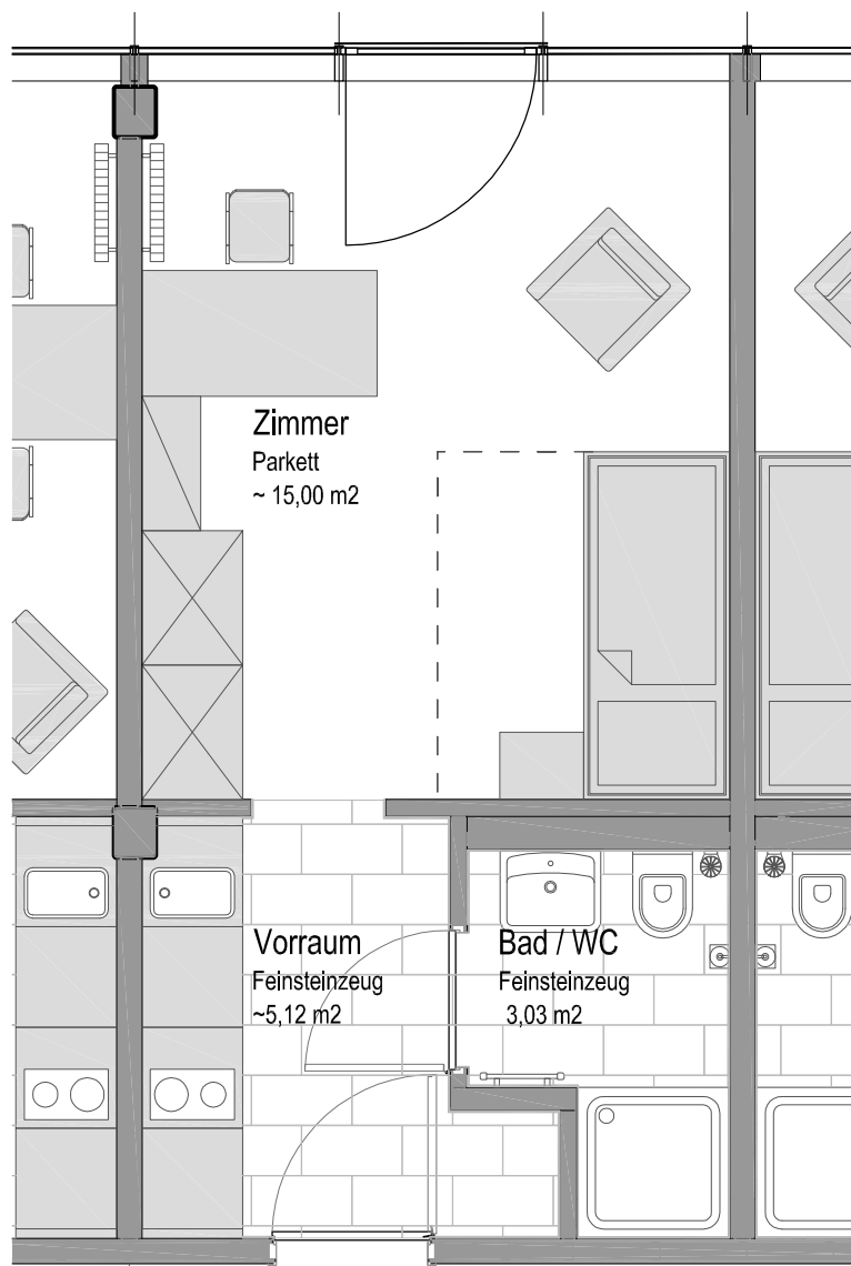
Grundriss M 1:50
