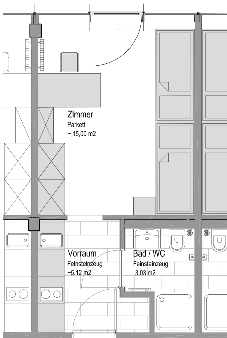
Grundriss M 1:50
