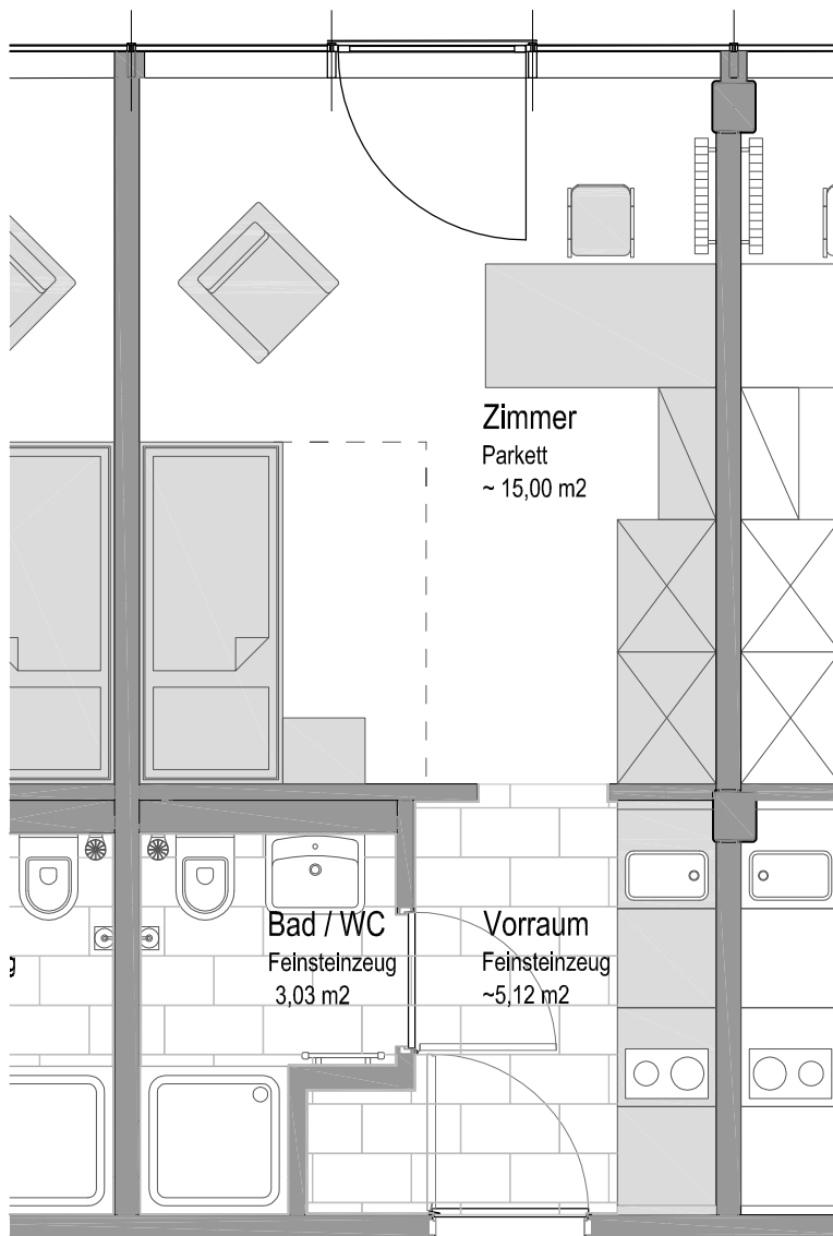
Grundriss M 1:50
